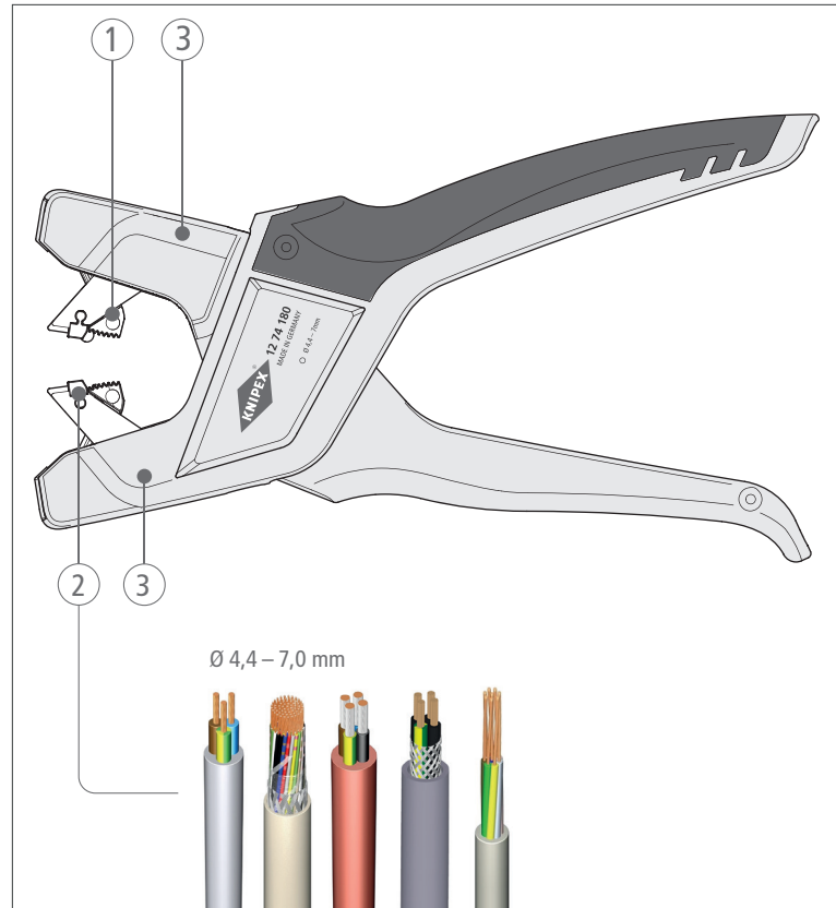
Estructura del pelacables multifuncional automático para cables redondos
