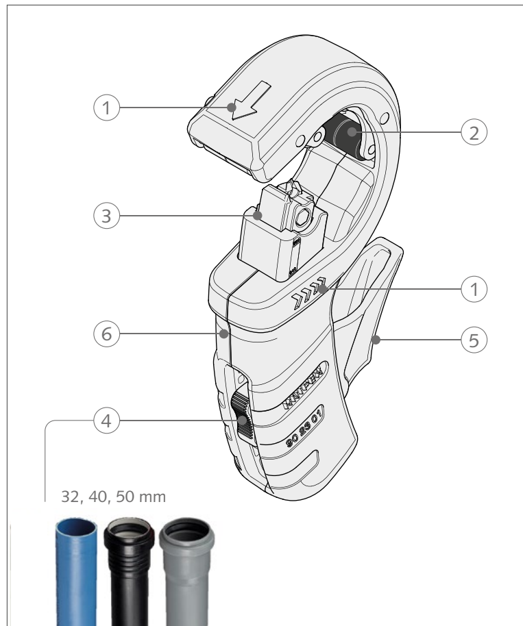
Aufbau Rohrabschneider DP50
