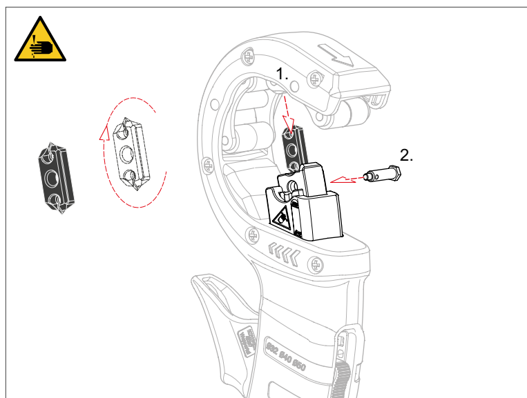
Klinge einsetzen
