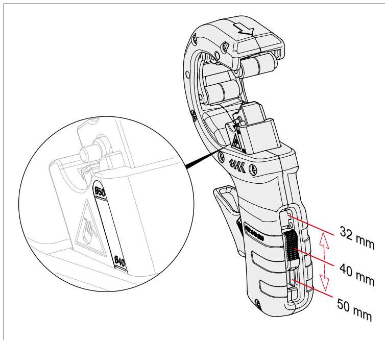
Einstellen des Werkzeugs auf den zu schneidenden Rohrdurchmesser
