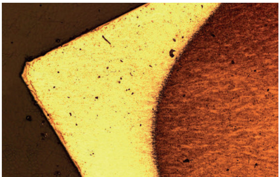
Makroaufnahme einer Schneide nach dem Induktivhärten. Präzise hebt sich der spezialgehärtete Schneidenbereich (hell) von der weicherer Gefügestruktur des Zangenkörpers (dunkel) ab.
