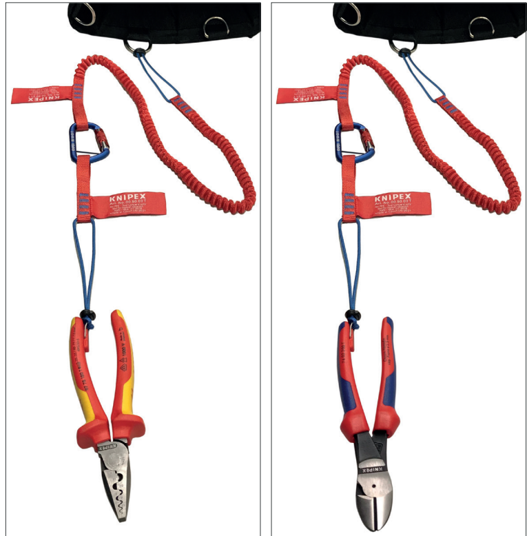
Abbildung 9: Anbringen von Adapterschlaufen
