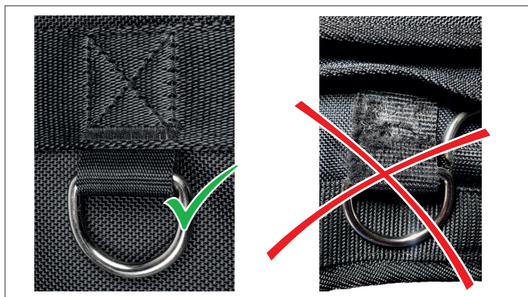
Abbildung 12: Die Nähte auf Beschädigungen überprüfen
