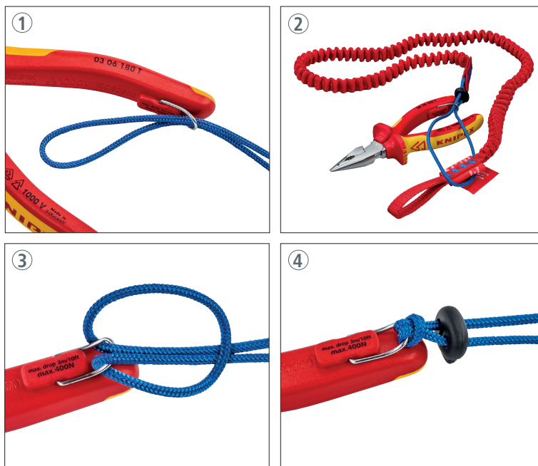
Figur 6: Tilkobling via løkke
