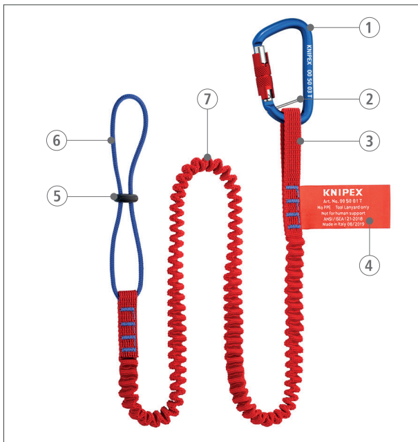
Figur 1: Begreper og definisjoner – festesnor, 1,5 kg (3,3 lbs)
