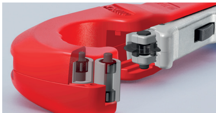
Des roulements à aiguilles de haute qualité permettent à la molette de coupe et aux quatre rouleaux de guidage de fonctionner pratiquement sans frottement gênant pendant la coupe – coupe les tubes en acier inoxydable avec une facilité extraordinaire
